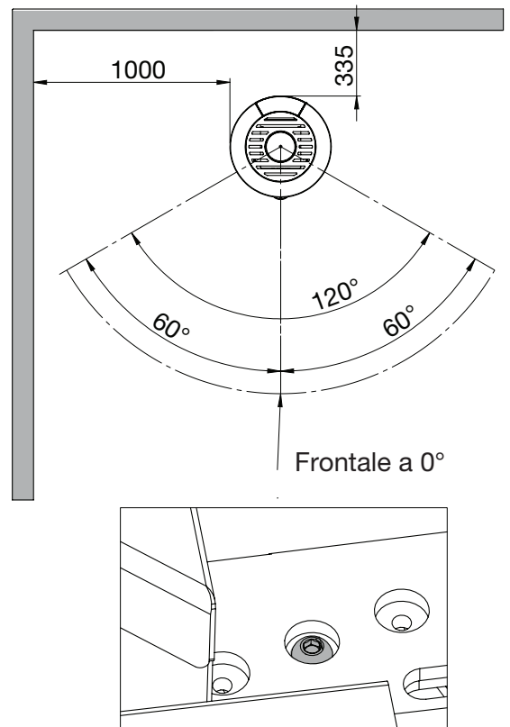
Base girevole bloccata a 120° e 60° su ciascun lato
